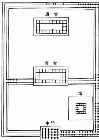
挿図3 大官大寺伽藍配置図 S 1 : 3000
