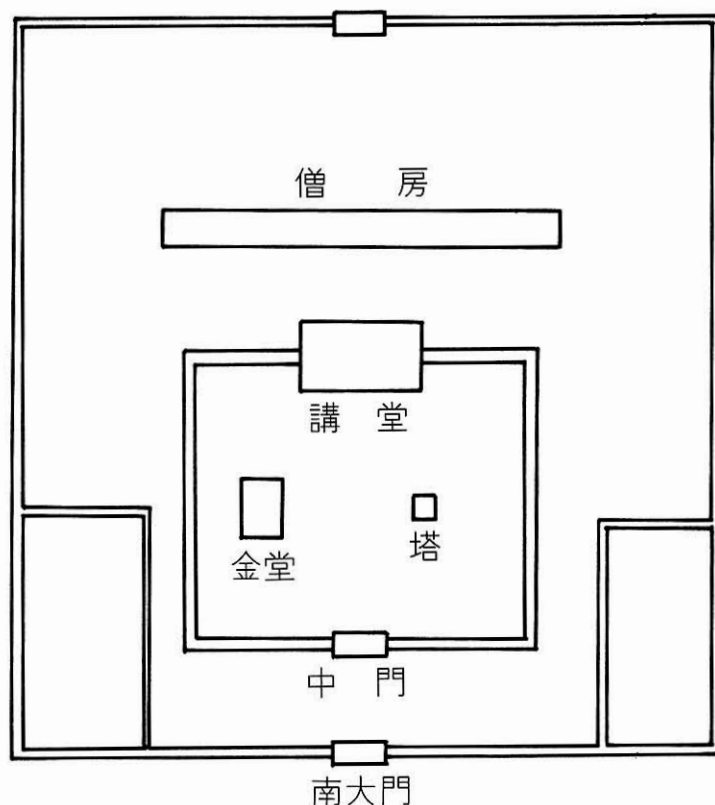
挿図2 観世音寺伽藍配置図 S 1 : 2000
